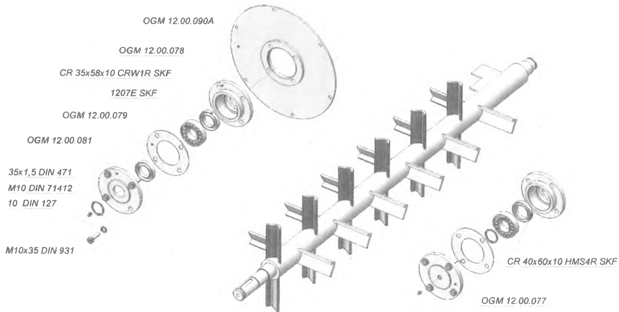
Pav. 10. Maišytuvas (OGM 12.00.000) Pic. 10. Distributor Рис. 10. Смеситель
