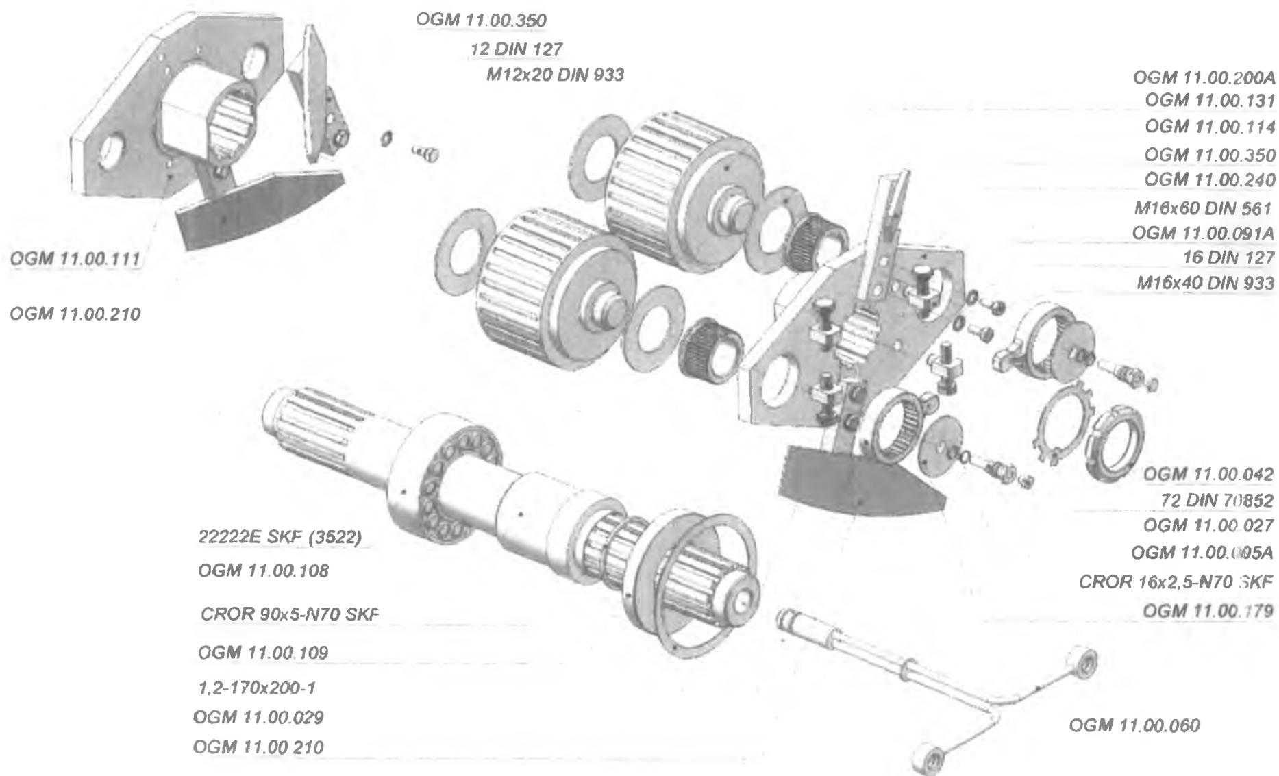
Pav. 3. Presas (OGM 11.00.000) Pic. 3. Press Рис. 3. Пресс
