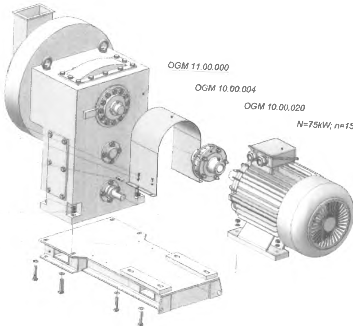
Рав. 1. Granulatorius (OGM 10.00.000) Pic. 1. Pelletizing equipment Рис. 1. Гранулятор
